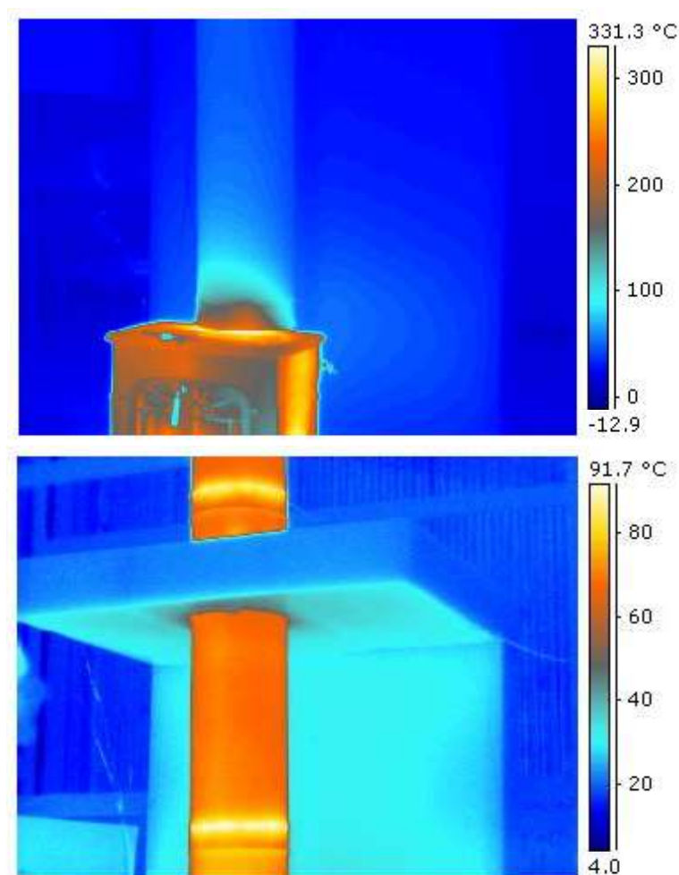
Figur 7: IR-bilder på kamin och skorsten, observera de två bilderna har olika temperaturskala. Observera också de varmare linjerna på skorstenen vid skarvarna. Vid detta försök monterades inte lasbandet runt skarven.
