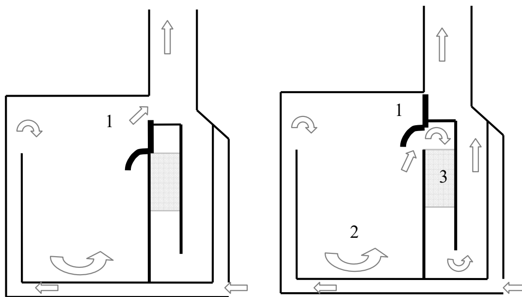
Figur 2: Schematisk bild över luft- och rökgasflödena i kaminen, förbränning utan katalysator och förbränning med katalysator. Den inkommande luften leds även i väggarna
