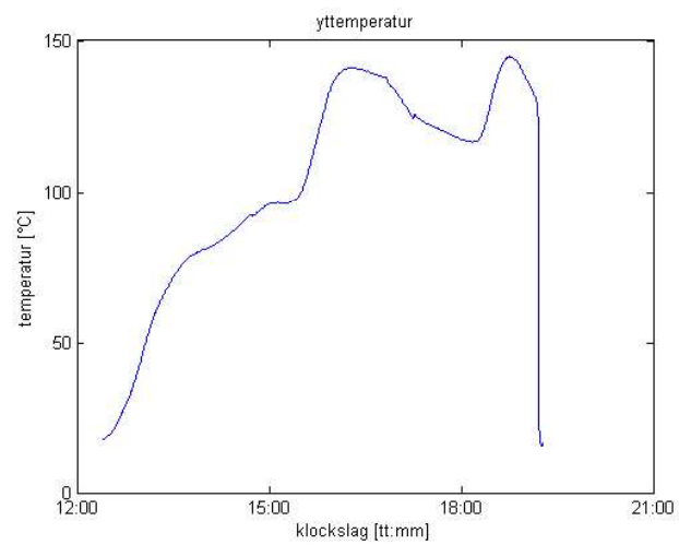
Figur 42: Temperaturen på skorstenens yta i schaktets topp
