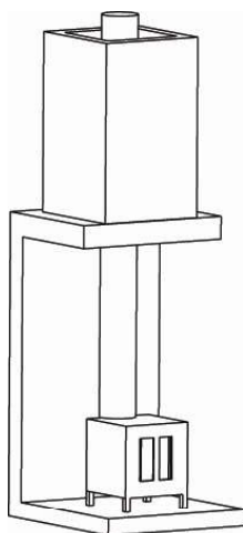
Figur 35: Schematisk bild över testriggen, med ett schakt monterat ovanpå taket.
