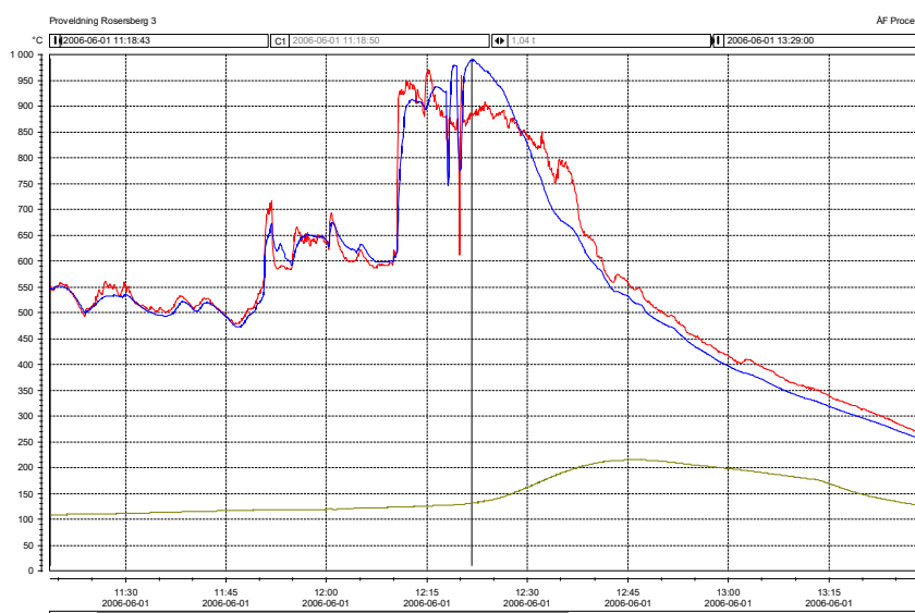
Figur 12. Rök-gastemperaturen (blå), kamintemperaturen (röd) och bjälklagsttemperaturen (grön) vid Försök 3. Figuren visar perioden för eldning med 50% överlast, öppning av förbigångsspjället samt avsvälningen..
