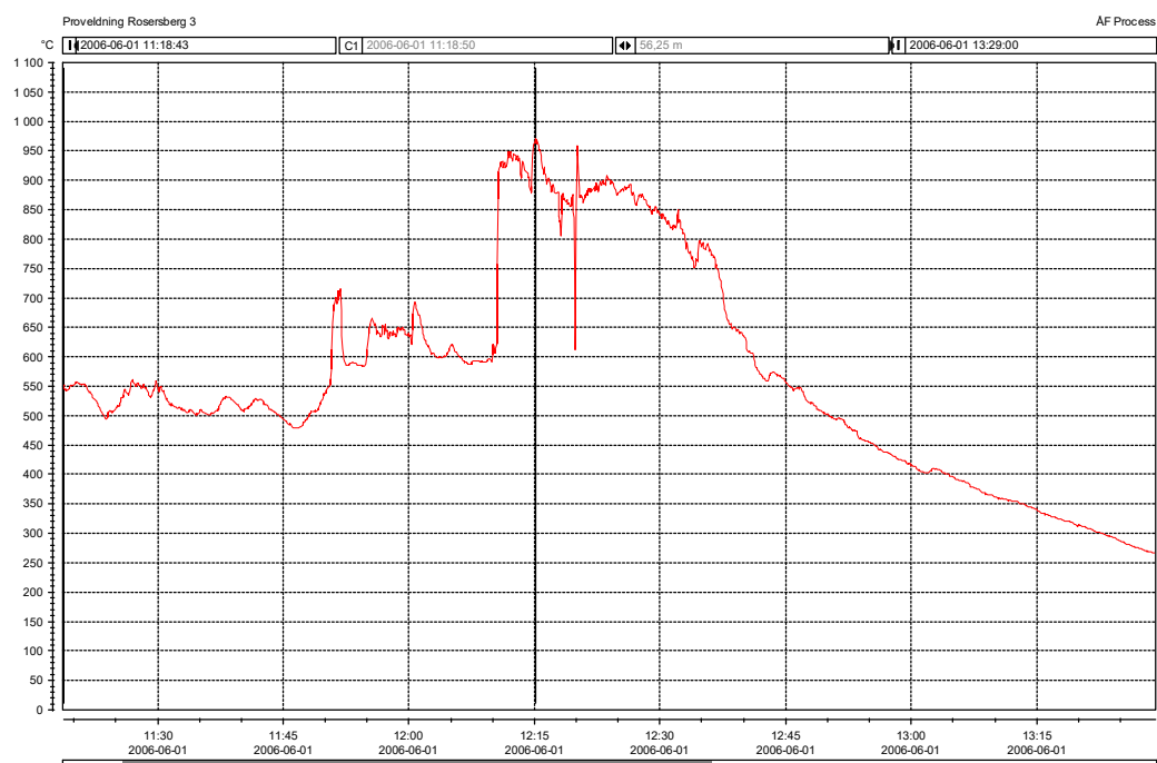
Figur 43: Kamintemperatur i samband med den tredje eldningen
