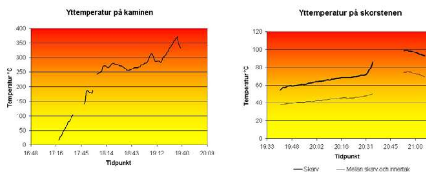
Figur 8: Maximala ytemperaturen som funktion av tiden på kamin och skorsten. Pga omflyttning av kamerans fokus så är signalen inte helt kontinuerlig.
