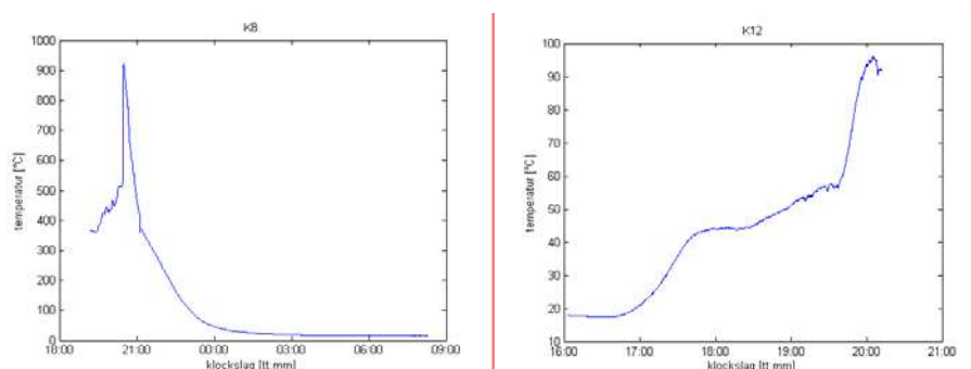
Figur 6: Temperatur som funktion av tiden. Givare K8 mäter rökgastemperaturen och givare K12 mäter på en punkt belägen mellan röret och isoleringen i taket. Observera de olika skalorna. Toppen erhöles när bypass spjället öppnades.
