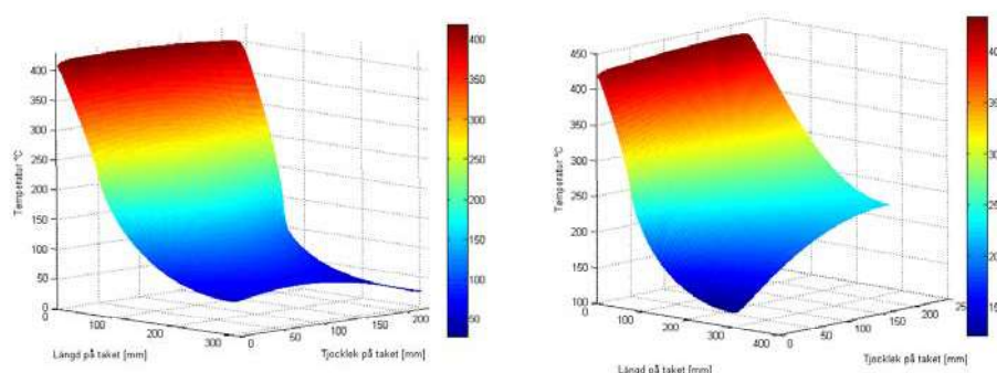
Figur 19: Temperaturvariation i tak och skorsten, med naturlig konvektion från taket till rummet (till vänster) och med övre delen av taket isolerad (till höger). Temperaturen på ovansidan av taket blir mycket varmare än temperaturen på undersidan, på grund av i
