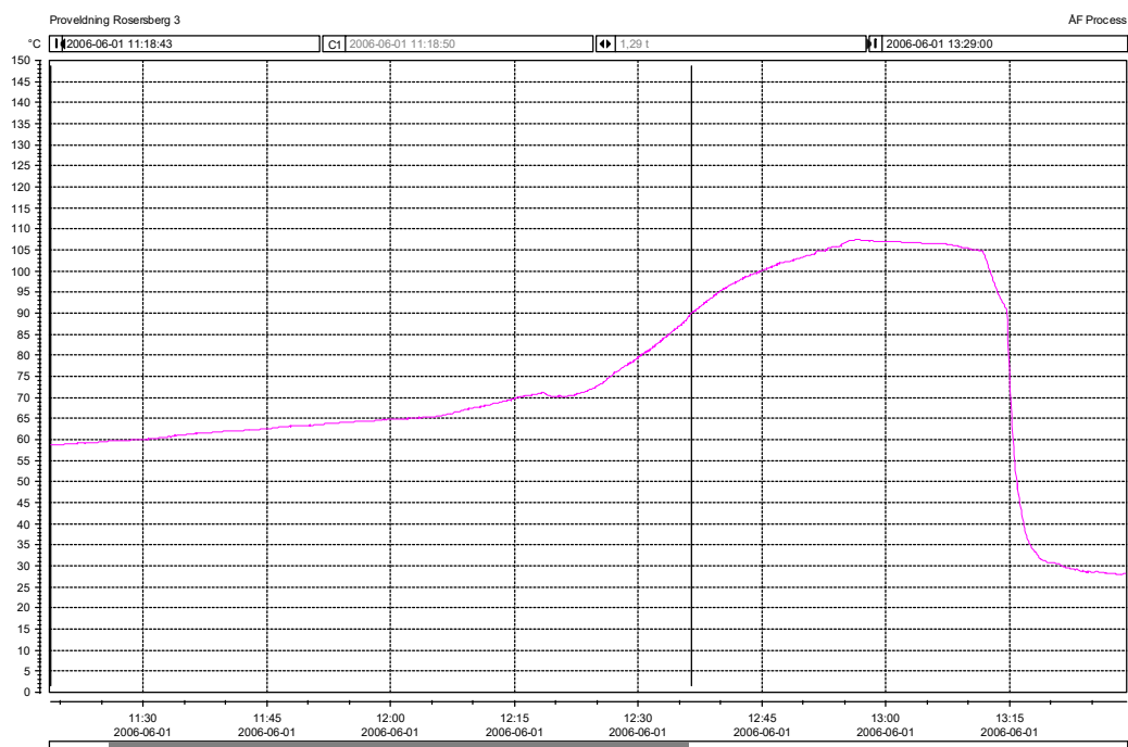
Figur 49: K15 Temperaturen i schaktet med termoelementet instuckat uppifrån.
